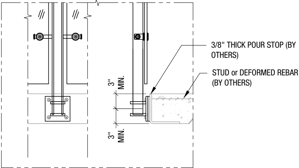
Welded @ Pour Stop - $$ Detail# BLA-F05
